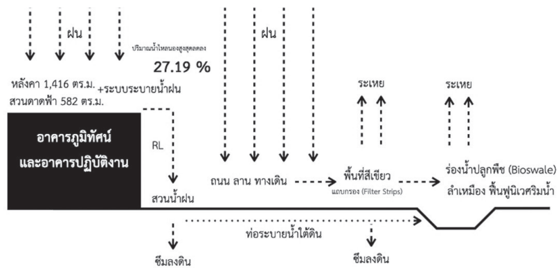
ภาพที่ 9 แนวคิดการจัดการน้ำฝนอาคารภูมิทัศน์และอาคารปฏิบัติงานระยะที่ 2
