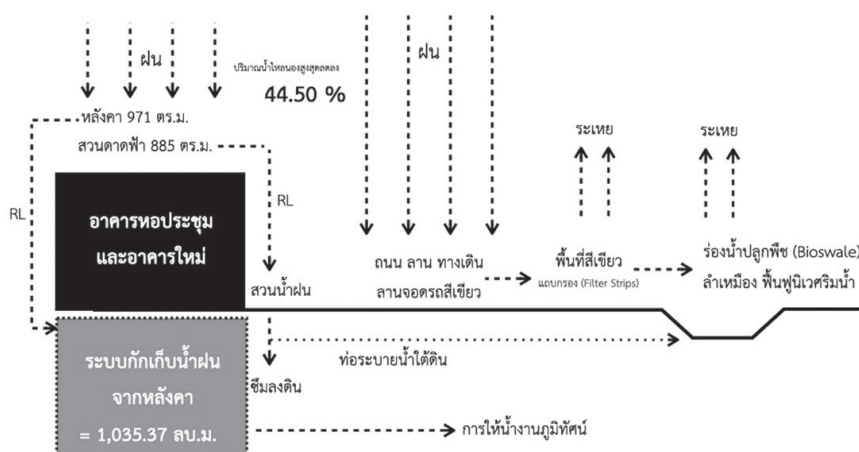
ภาพที่ 12 แนวคิดการจัดการน้ำฝนอาคารเรียนคณะสถาปัตยกรรมศาสตร์ฯ (อาคารใหม่) และอาคารหอประชุมระยะที่ 3
