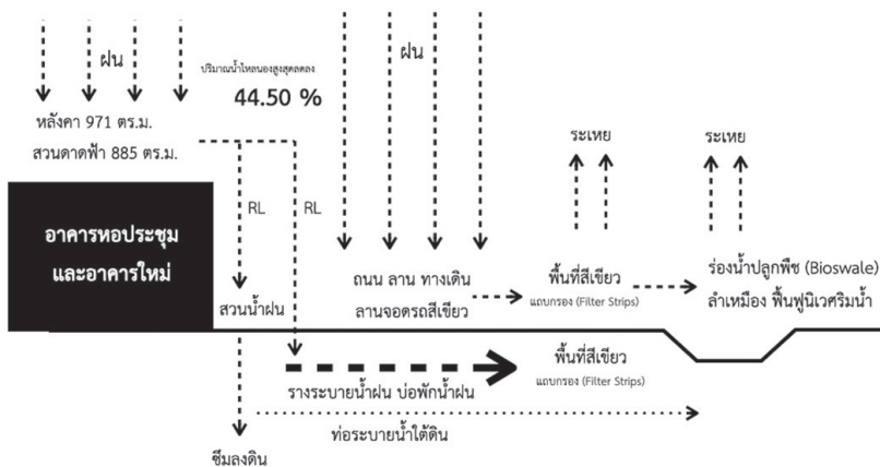
ภาพที่ 10 แนวคิดการจัดการน้ำฝนอาคารเรียนคณะสถาปัตยกรรมศาสตร์ฯ (อาคารใหม่) และอาคารหอประชุมระยะที่ 2
