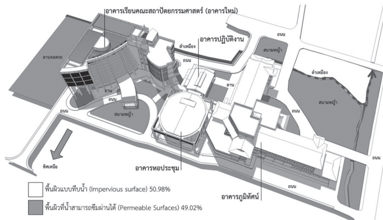
ภาพที่ 2 ลักษณะทางกายภาพของสถาปัตยกรรมศาสตร์ฯ และประเภทสิ่งปกคลุมดินที่ส่งผลต่อการซึมน้ำ
