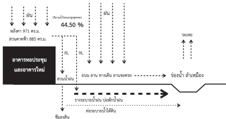
ภาพที่ 8 แนวคิดการจัดการน้ำฝนอาคารเรียนคณะสถาปัตยกรรมศาสตร์ฯ (อาคารใหม่) และอาคารหอประชุมระยะที่ 1
