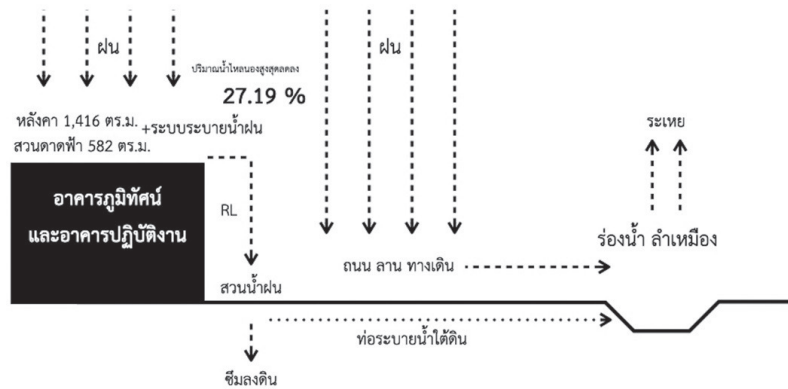
ภาพที่ 7 แนวคิดการจัดการน้ำฝนอาคารภูมิทัศน์และอาคารปฏิบัติงานระยะที่ 1
