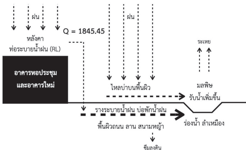
ภาพที่ 6 สรุปข้อมูลการจัดการน้ำฝนและปัญหาสำหรับอาคารที่มีระบบจัดการน้ำฝน
