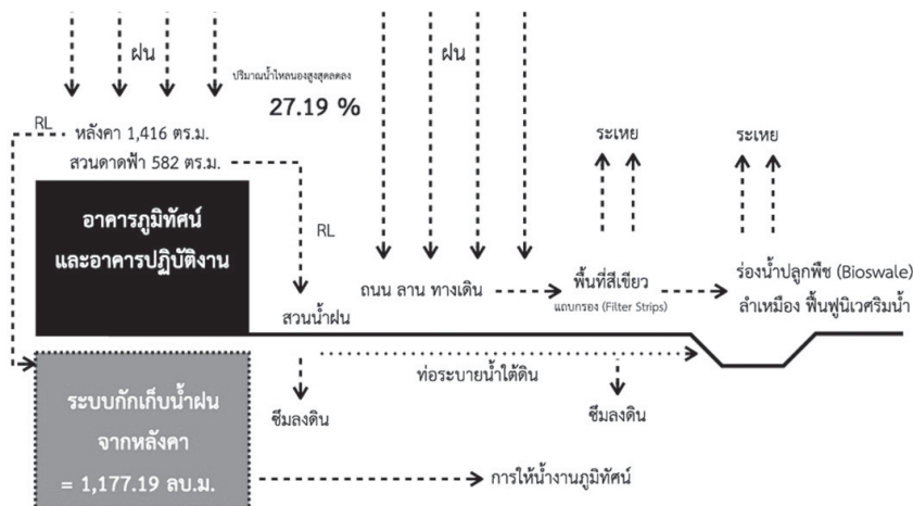
ภาพที่ 11 แนวคิดการจัดการน้ำฝนอาคารภูมิทัศน์และอาคารปฏิบัติงานระยะที่ 3
