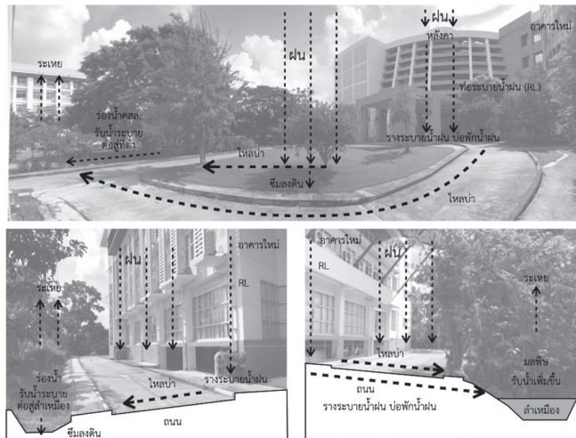
ภาพที่ 4 การจัดการน้ำฝนและสภาพปัญหาของอาคารหอประชุม และอาคารเรียนคณะสถาปัตยกรรมศาสตร์ฯ
