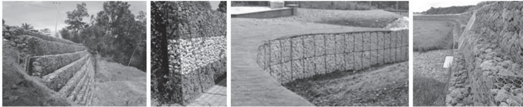
ภาพที่ 10 กล่องกระชุน หรือกล่องลวดตาข่าย (Landscapingnetwork, 2019)
