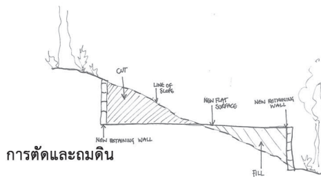
ภาพที่ 8 การปรับแก้สภาพภูมิประเทศ โดยการตัดและถมดินเพื่อให้ได้ระดับที่ต้องการ (Sterlingcodifiers.com, 2019)
