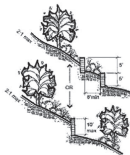
ภาพที่ 9 การปรับแก้สภาพภูมิประเทศ โดยใช้กำแพงกันดินเพื่อให้ได้ระดับที่ต้องการ (Sterlingcodifiers.com, 2019)
