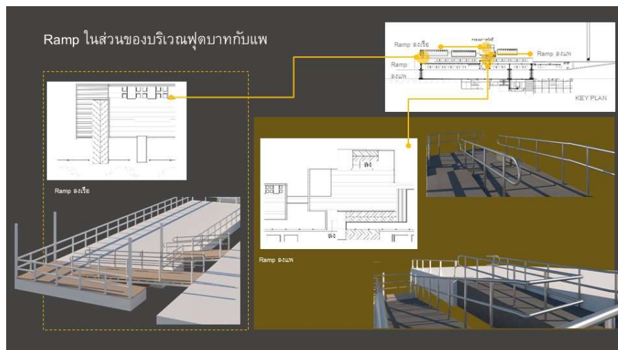
ภาพ 6 แนวทางการออกแบบพัฒนา นำเสนอภาพ 3 มิติ ท่าเรือ (จุดขึ้นลงเรือ)
