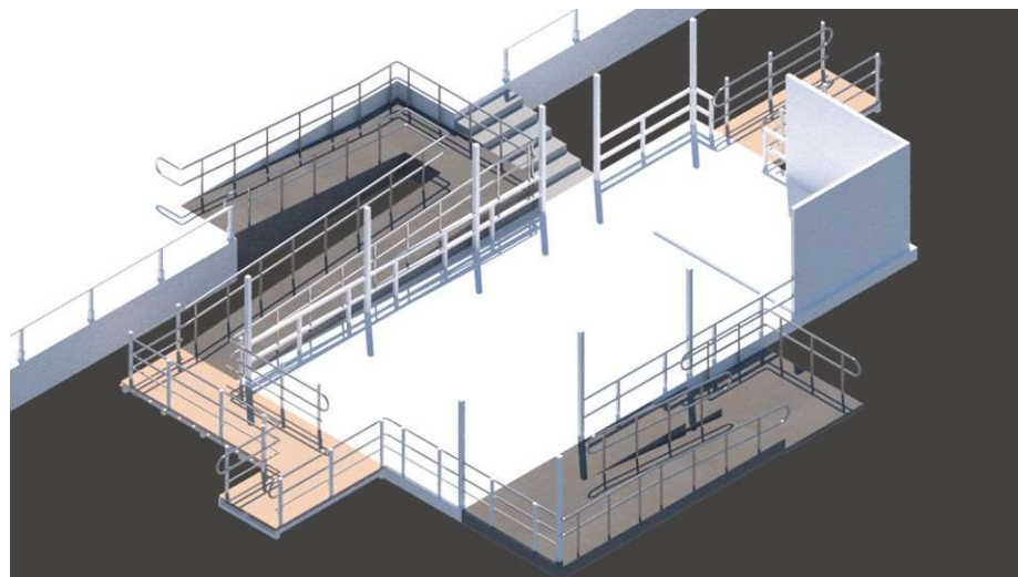
ภาพ 8 แนวทางปรับปรุงท่าเรือ (จุดขึ้นลงเรือ) สำหรับคนพิการและผู้สูงอายุ ตลาดน้ำบ้านศาลาดิน
