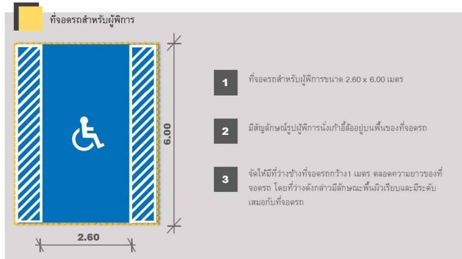
ภาพ 16 แนวทางการปรับปรุงจุดจอดรถให้มีขนาดเหมาะสม มีสัญลักษณ์ สำหรับคนพิการและผู้สูงอายุ
