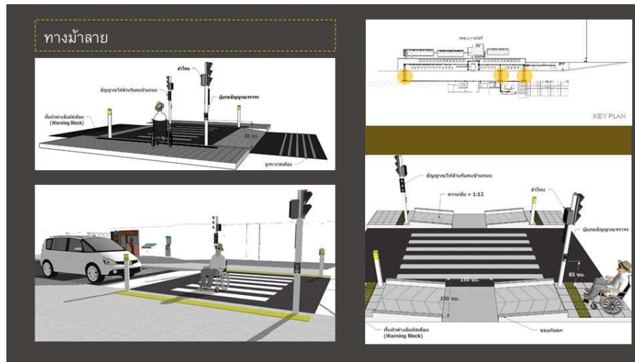
ภาพ 5 แนวทางการออกแบบพัฒนา นำเสนอภาพ 3 มิติ ทางม้าลายจุดข้ามถนน ความลาดชัน (Slope) และสัญญาณไฟจราจร
