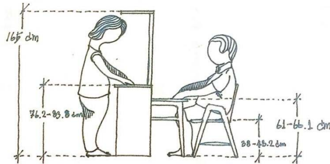
ภาพ 2 แสดงระยะความสูงส่วนต่างๆ ของชุดครัวที่เหมาะสมกับผู้สูงอายุจากการวิเคราะห์ด้วยข้อมูลการลงพื้นที่สำรวจ
