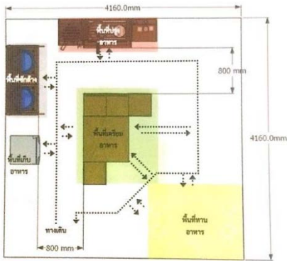
ภาพ 12 ตัวอย่างเบื้องต้นพื้นที่เตรียมอาหารที่สามารถปรับเปลี่ยนรูปแบบได้
