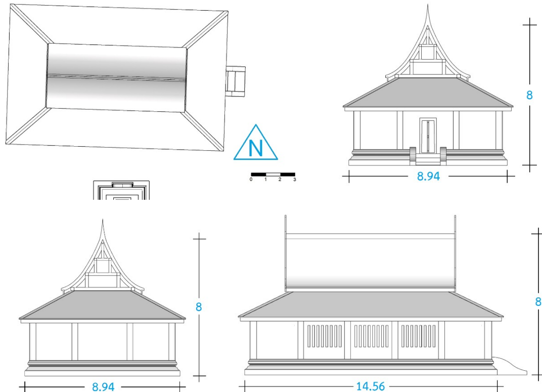
ภาพ 25 ภาพสันนิษฐาน แผนผัง รูปด้านทิศตะวันออก ทิศตะวันตก และทิศใต้ พระอุโบสถ หรือพระวิหารราย ที่มา : อนัสพงษ์ ไกรเกรียงศรี
