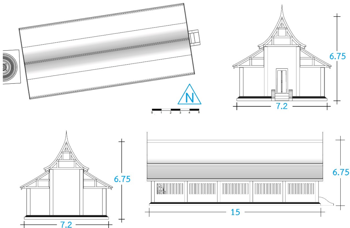
ภาพ 10 ภาพสันนิษฐาน แผนผัง รูปด้านทิศตะวันออก ทิศตะวันตก และทิศใต้ พระวิหารหลวง ที่มา: อนัสพงษ์ ไกรเกรียงศรี
