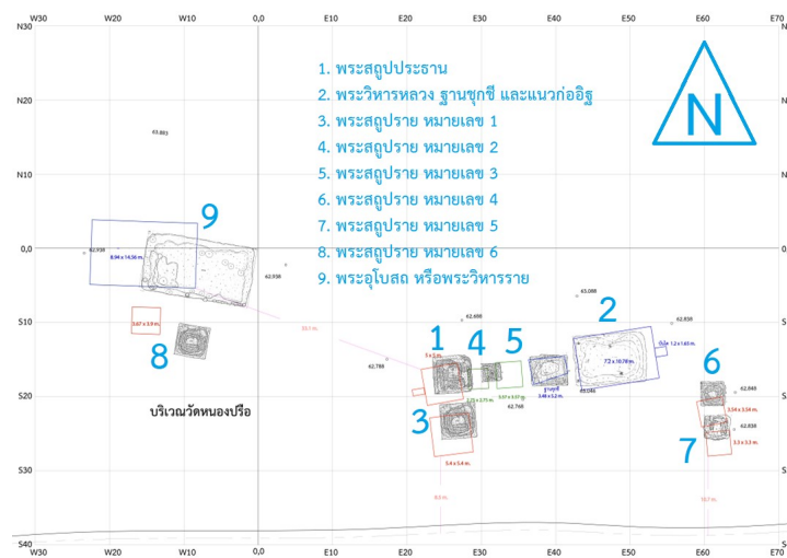
ภาพ 4 ผังบริเวณโบราณสถานวัดหนองปรือ และแนวชุดสำรวจ ที่มา: กรมศิลปากร, 2562
