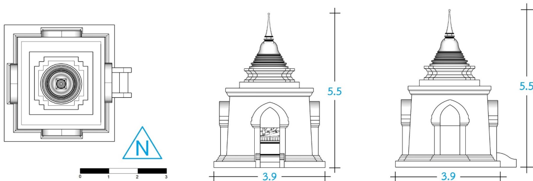
ภาพ 23 ภาพสันนิษฐาน แผนผัง รูปด้านทิศตะวันออก และทิศใต้ พระสถูปราย หมายเลข 6 ที่มา : อนัสพงษ์ ไกรเกรียงศรี
