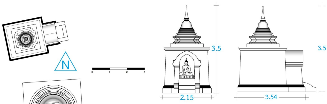
ภาพ 19 ภาพสันนิษฐาน แผนผัง และรูปด้านทิศตะวันออกเฉียงใต้ และทิศใต้ พระสถูปราย หมายเลข 4 ที่มา: อนัสพงษ์ ไกรเกรียงศรี
