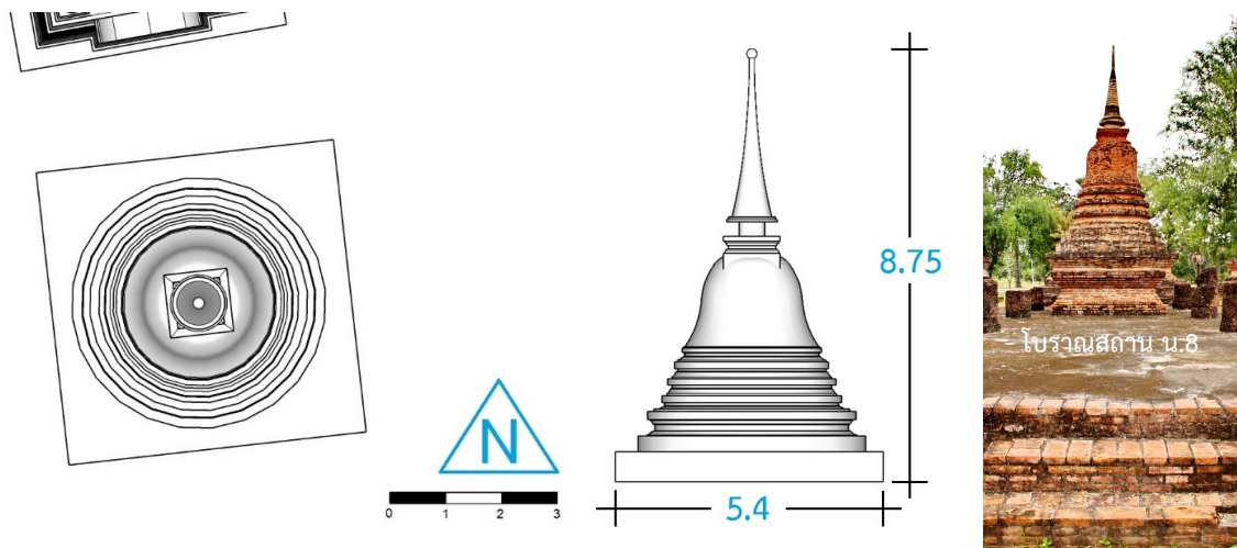
ภาพ 13 ภาพสันนิษฐาน แผนผัง และรูปด้านทิศตะวันออก พระสถูปราย หมายเลข 1 และพระสถูปทรงระฆังที่โบราณสถาน หมายเลข น. 8 ที่มา : อนัสพงษ์ ไกรเกรียงศรี
