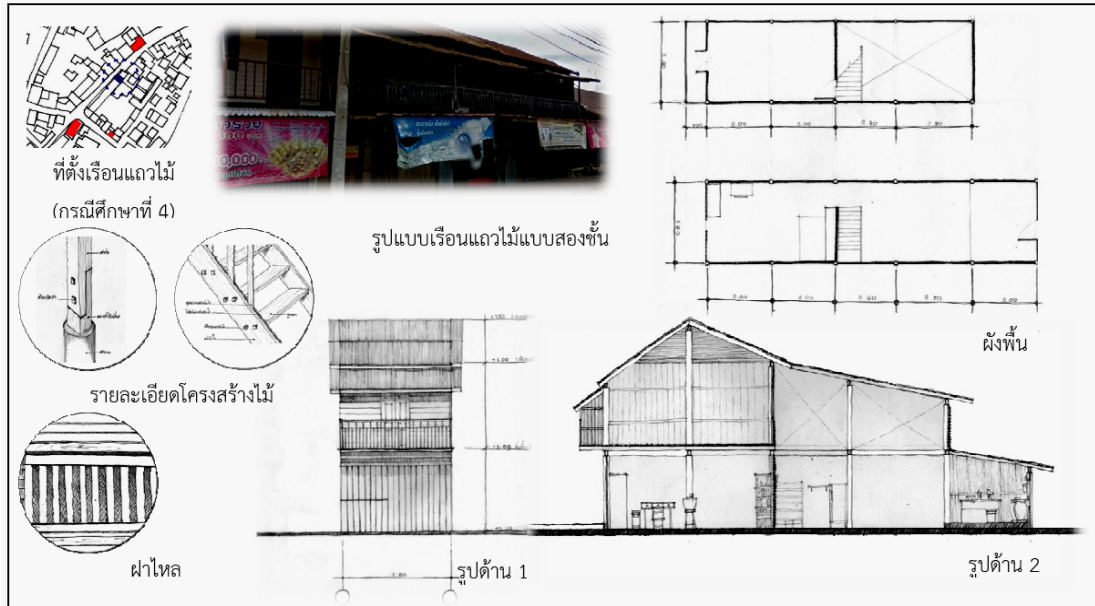
ภาพ 5 เรือนแถวไม้แบบสองชั้นกรณีศึกษาที่ 4 พื้นที่หลังเรือนแถวชั้นล่าง-บนเปิดโล่ง
