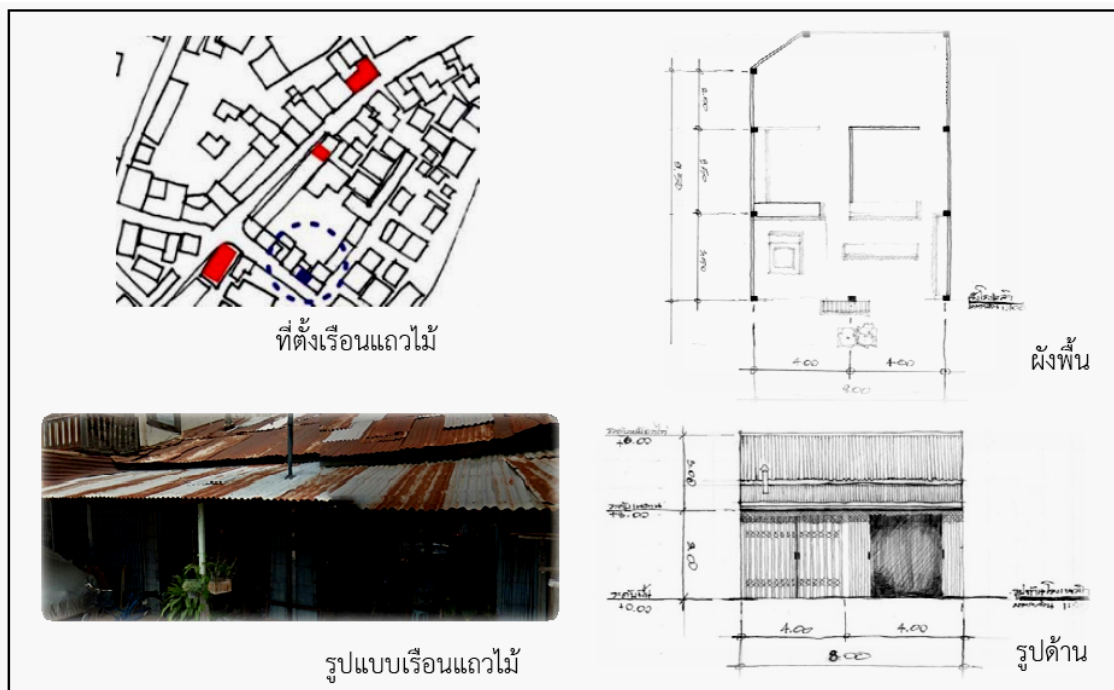
ภาพ 4 เรือนแถวไม้แบบชั้นเดียวกรณีศึกษาที่ 3 มีการเปิดพื้นที่ภายใน และจัดห้องน้ำไว้ด้านนอก
