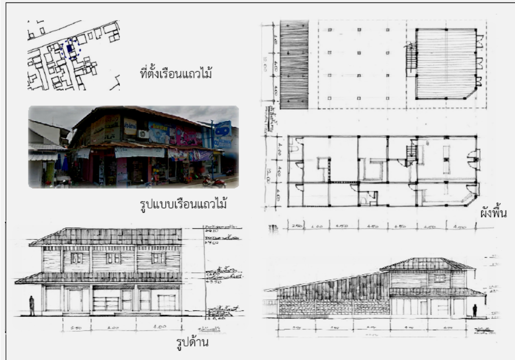
ภาพ 7 เรือนแถวไม้หัวมุมถนนแบบสองชั้นกรณีศึกษาที่ 6 มีการกันห้องจากเดิมที่เปิดโล่ง
