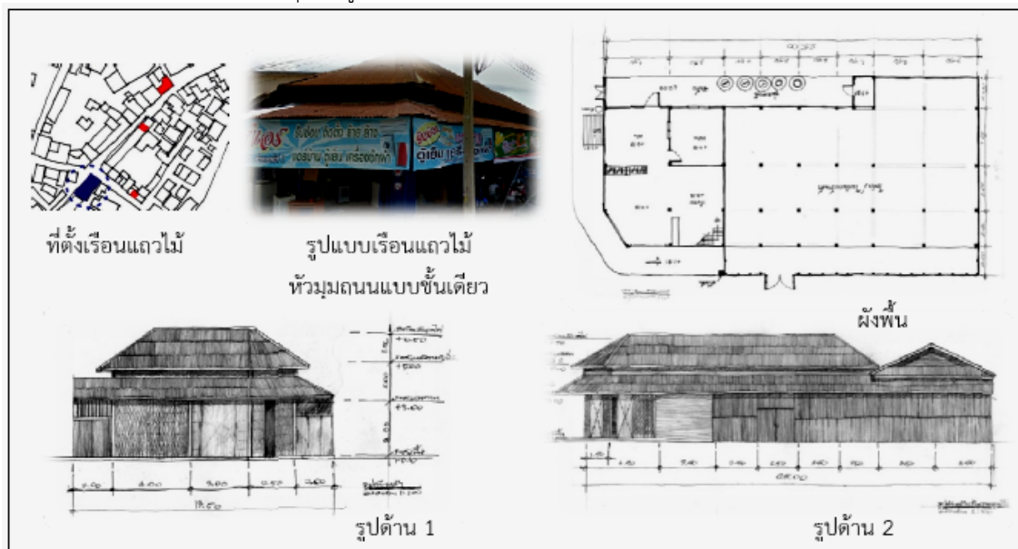
ภาพ 6 เรือนแถวไม้หัวมุมถนนแบบชั้นเดียวแบบสองชั้นกรณีศึกษาที่ 5 หลังคาแบบผสม
