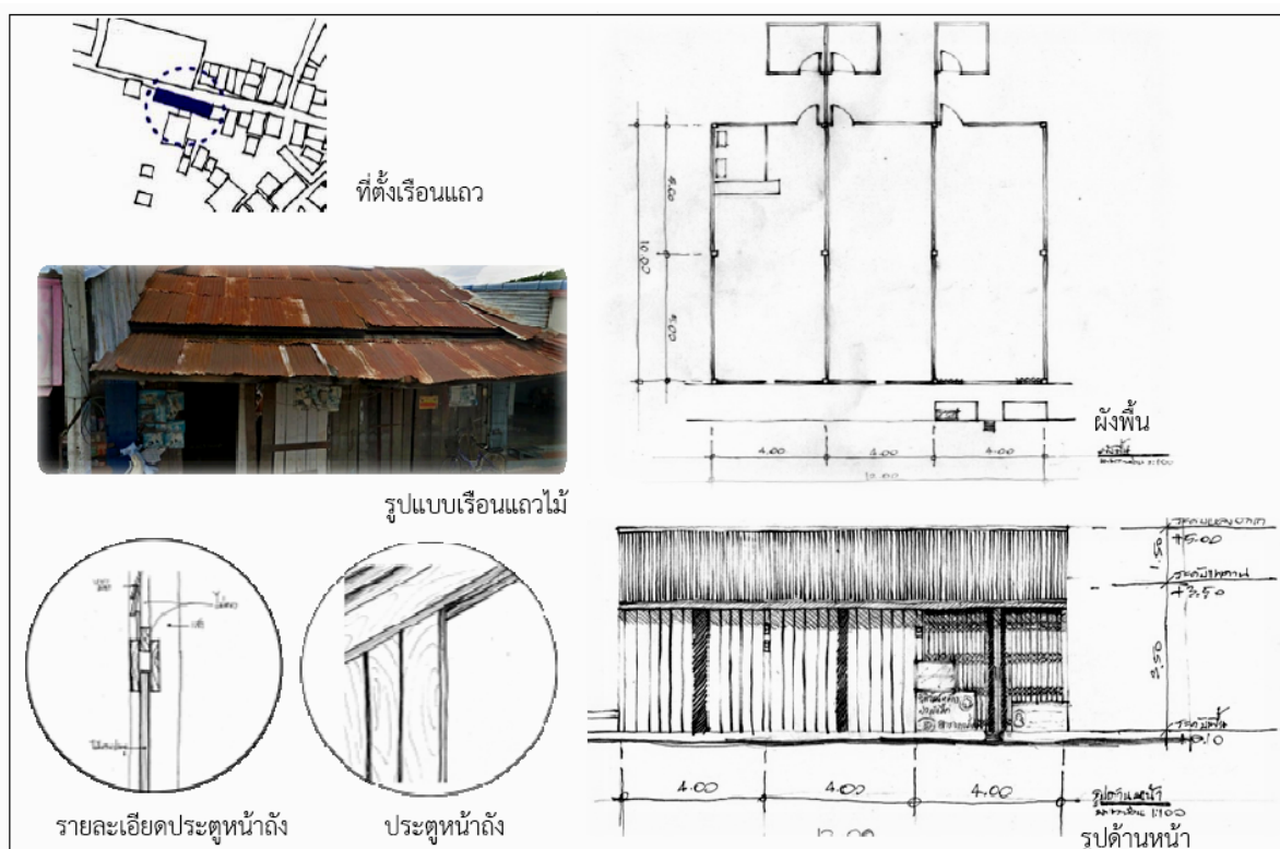
ภาพ 2 เรือนแถวไม้แบบชั้นเดียวกรณีศึกษาที่ 1 มีการเปิดพื้นที่ภายใน และจัดให้มีห้องน้ำไว้ด้านนอก
