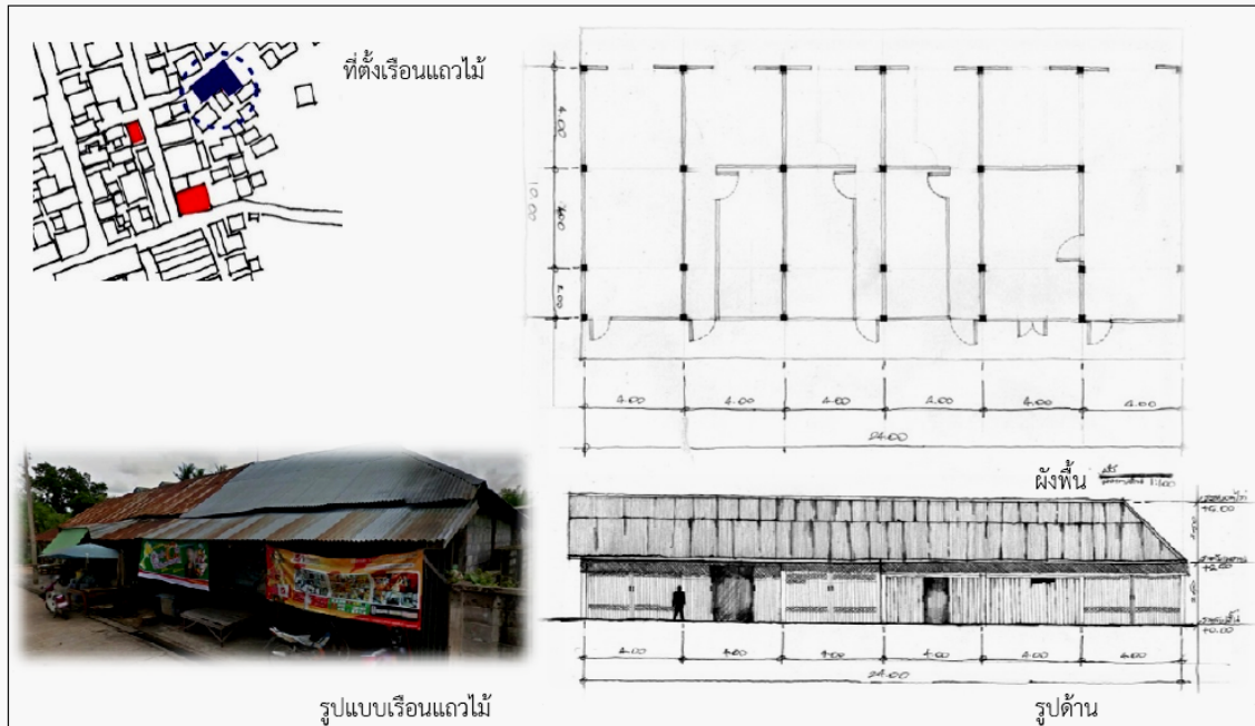
ภาพ 3 เรือนแถวไม้แบบชั้นเดียวกรณีศึกษาที่ 2 มีการกันห้องภายใน แต่เกิดขึ้นภายหลัง
