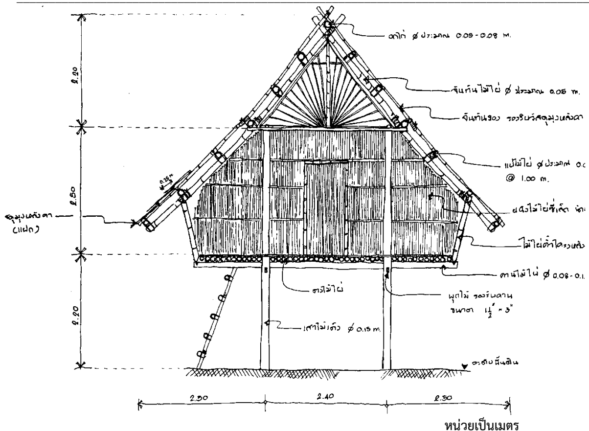
ภาพ ๗ รูปตัดแสดงรายละเอียดโครงสร้างของเรือน (ที่มา: คณะผู้วิจัย)
