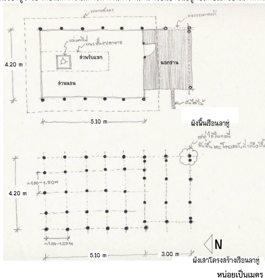
ภาพ ๓ ภาพวาดผังเรือนและโครงสร้างเสาเรือนลาหู่ อำเภอเมือง จังหวัดตาก (ที่มา: คณะผู้วิจัย)
