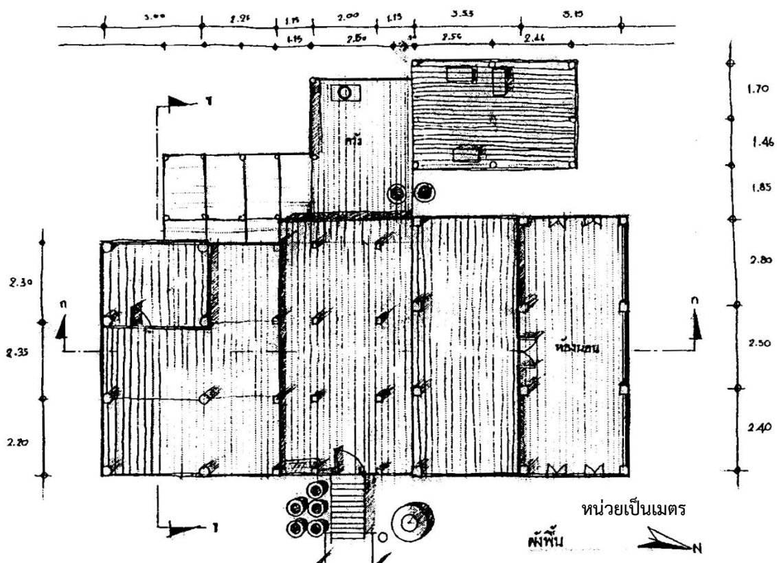
ภาพ ๙ ผังพื้นเรือน บ้านไผ่ขื่อน้ำ อำเภอพรหมพิราม จังหวัดพิษณุโลก (ที่มา: คณะผู้วิจัย)
