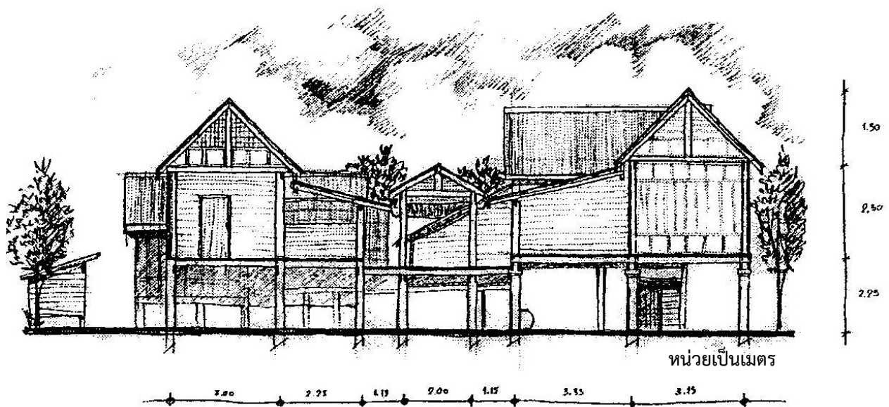
ภาพ ๑๐ รูปตัดเรื่อนตามยาว บ้านไผ่ขื่อน้ำ อำเภอรพรมพิราม จังหวัดพิษณุโลก (ที่มา: คณะผู้วิจัย)
