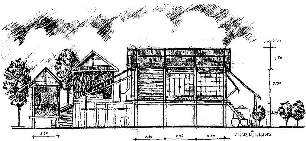
ภาพ ๑๑ รูปตัดเรื่อนตามขวาง บ้านไผ่ขื่อน้ำ อำเภอรพรมพิราม จังหวัดพิษณุโลก (ที่มา: คณะผู้วิจัย)
