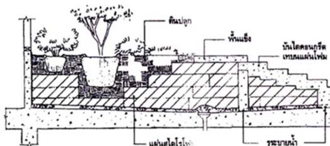
ภาพ 14 แสดงการใช้สไตรโฟมหนุนด้านล่างเพื่อลดปริมาณวัสดุปลูกหรือดินปลูก ที่มา : จามรี อารยานิมิตสกุล 2535.
