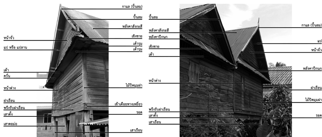
ภาพที่ 5 แสดงส่วนประกอบและเทคนิคก่อสร้างของเรือนกรณีศึกษาที่ 1 (ซ้าย) และ 3 (ขวา) มุมมองด้านสกัดข้าง หลังเรือน
