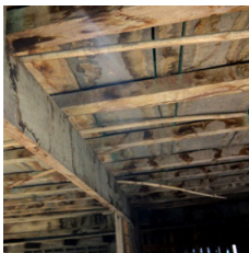
การวางตงแนวนอนแบบดั้งเดิม
