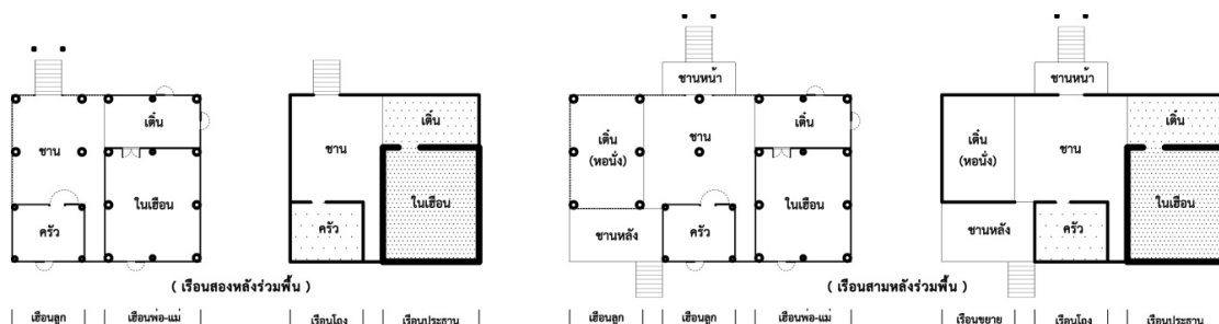
ภาพที่ 4 แสดงตัวอย่างผังพื้นดั้งเดิมและแบบแผนพื้นที่ใช้สอยของเรือนยวนสี่คี่
