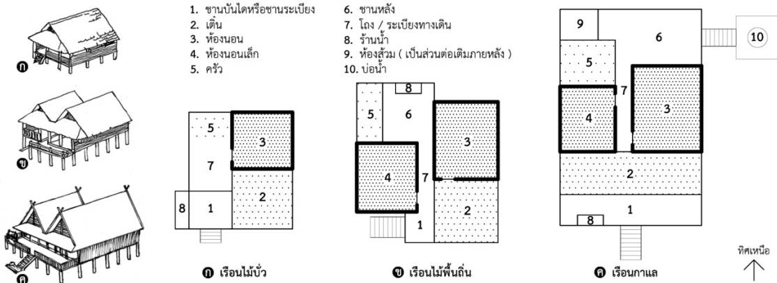
ภาพที่ 1 แสดงรูปแบบของเรือนไทยในภาคเหนือ (ก) เรือนไม้บัว (ข) เรือนไม้พื้นถิ่น และ (ค) เรือนกาแล ที่มา: คัดลอกจากข้อมูลของ อัน (2521 : 146-147) อนุวิทย์ (2539 : 9-10) และ สมคิด (2543 : 160)
