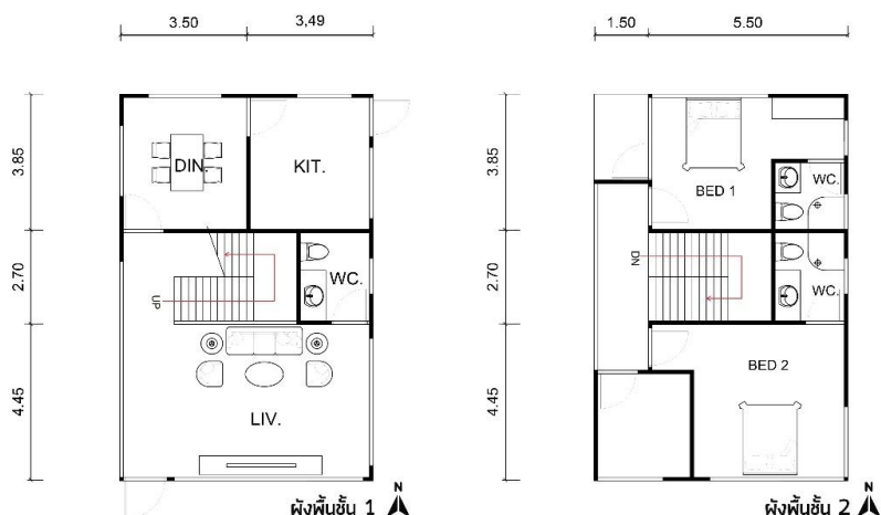
ภาพที่ 1 แสดงแบบผังบ้านพักอาศัยที่ออกแบบจากข้อมูลโครงการศึกษาเกณฑ์การใช้พลังงานในบ้านพักอาศัย และสร้างบ้านเพื่อการประหยัดพลังงาน พ.ศ.2559-2560
