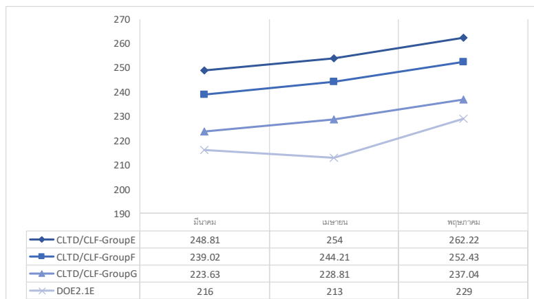
ภาพที่ 3 แผนภูมิแสดงการเปรียบเทียบค่าภาระการทำความเย็นจากการคำนวณด้วยวิธี CLTD/CLF กับการคำนวณโดยการจำลองด้วยระบบโปรแกรม DOE2.1E ver.121
