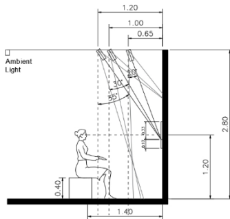
ภาพที่ 2 แสดงตำแหน่งการติดตั้งดวงโคมส่องสว่าง และตำแหน่งการรับชมภาพจัดแสดง
