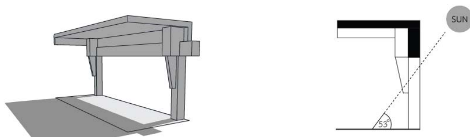
ภาพที่ 6 ตำแหน่งดวงอาทิตย์ในเดือนธันวาคม เวลา 12:00 น. ที่มุมอัลติจูดสูงสุด 53 องศา
