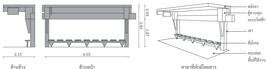
ภาพที่ 1 ขนาดและลักษณะของศาลาที่พักผู้โดยสารรถประจำทางแบบที่มีเฉพาะหลังคา
