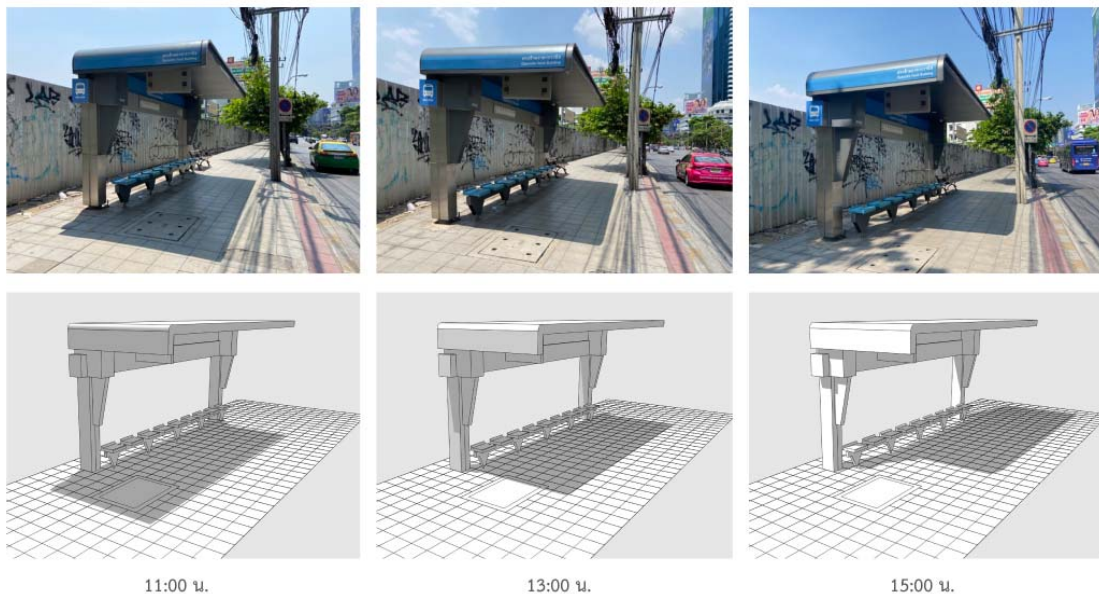
ภาพที่ 3 ลักษณะและรูปร่างของเงาจากศาลาที่เกิดขึ้นจริงกับแบบการจำลองเงาในโปรแกรม SketchUp
