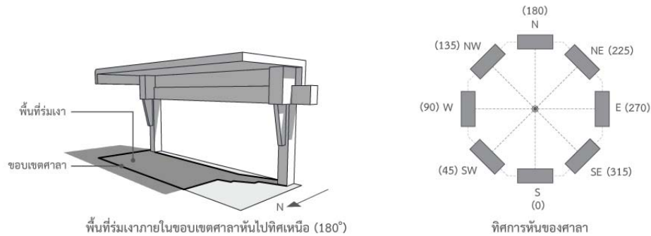
ภาพที่ 4 พื้นที่ร่มเงาภายในขอบเขตพื้นที่ศาลาและทิศทางการวางศาลาทั้ง 8 ทิศ
