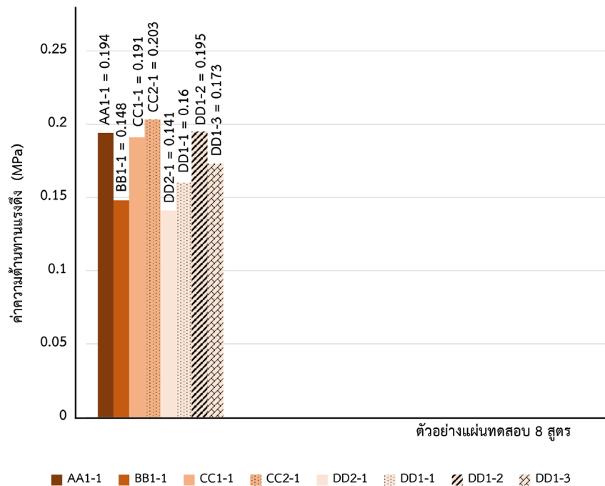
ภาพที่ 6 ค่าความต้านทานแรงดัดในอัตราส่วนต่าง ๆ ของแผ่นทดสอบ
