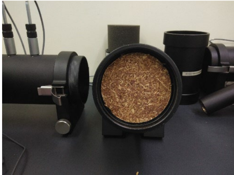
ภาพที่ 7 การทดสอบด้านการดูดซับเสียง แผ่นชิ้นงานที่ทดสอบ เส้นผ่าศูนย์กลาง 10 เซนติเมตร หนา 1 เซนติเมตร
