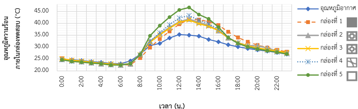
ภาพที่ 11 อุณหภูมิความร้อนภายในกล่องทดสอบทั้ง 5 กล่อง เป็นเวลา 24 ชม. ของการทดสอบครั้งที่ 1
