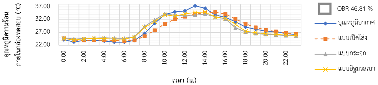
ภาพที่ 17 อุณหภูมิความร้อนภายในกล่องทดสอบทั้ง 3 กล่อง ที่มีบล็อก OBR 46.81 % เป็นผนังชั้นที่สองของการทดสอบชุดที่ 3.2
