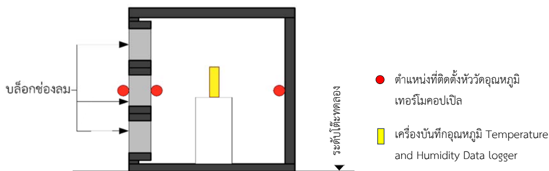
ภาพที่ 6 ตำแหน่งการวัดอุณหภูมิภายนอก และภายในกล้องทดสอบครั้งที่ 2
