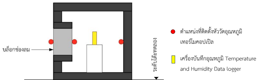
ภาพที่ 4 ตำแหน่งการวัดอุณหภูมิภายนอก และภายในกล่องทดสอบครั้งที่ 1
