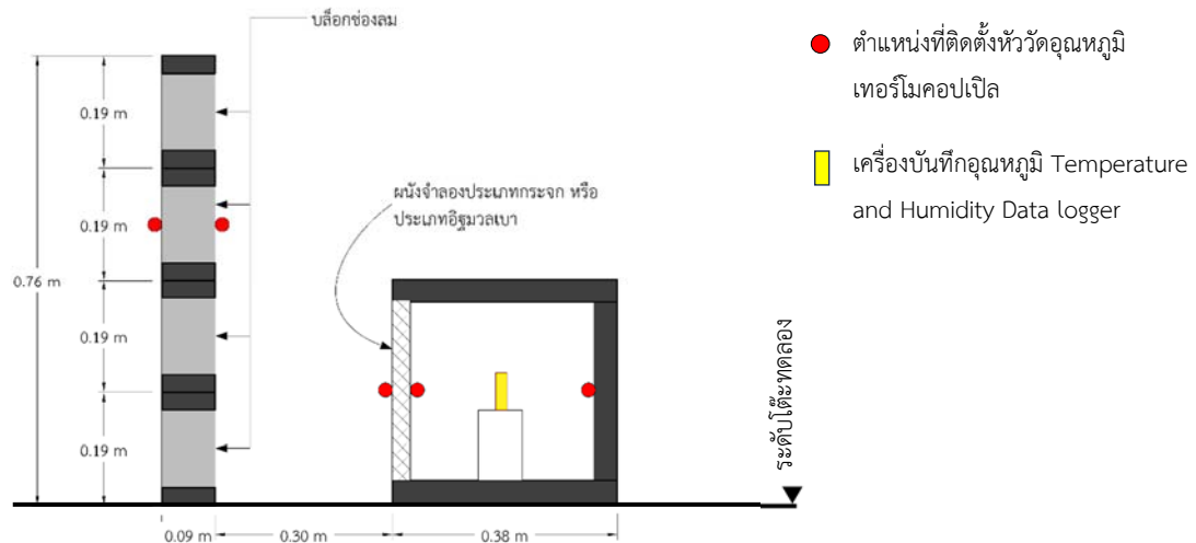
ภาพที่ 10 ตำแหน่งการวัดอุณหภูมิภายนอก และภายในกล่องทดสอบของผลการศึกษาการทดสอบครั้งที่ 3.2 และ 3.3
