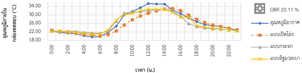
ภาพที่ 19 อุณหภูมิความร้อนภายในกล่องทดลองทั้ง 3 กล่อง ของการทดสอบชุดที่ 3.3
