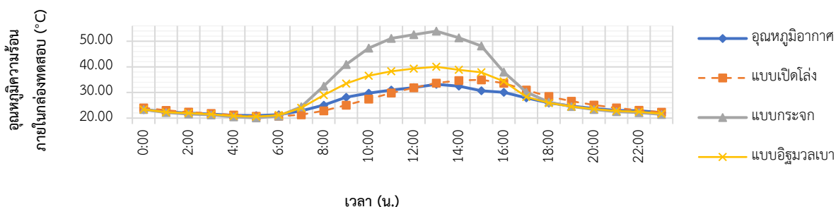
ภาพที่ 15 อุณหภูมิความร้อนภายในกล่องทดลองทั้ง 3 กล่อง ของการทดสอบชุดที่ 3.1
