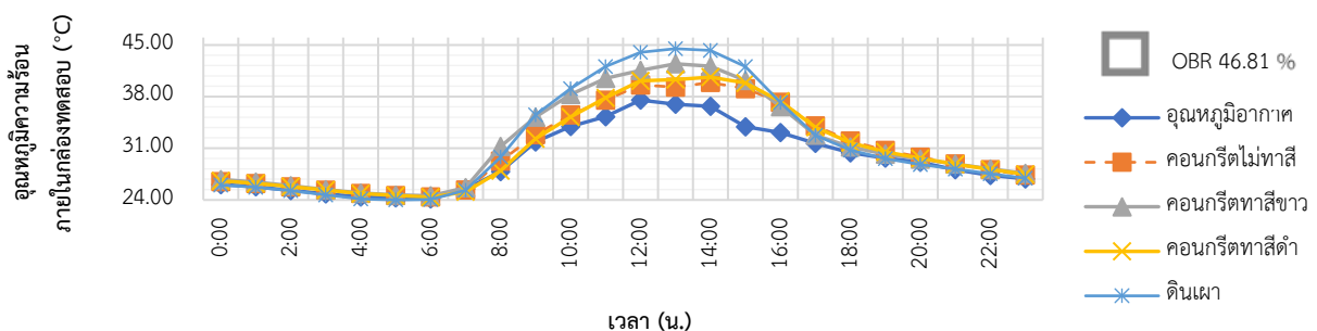
ภาพที่ 13 อุณหภูมิความร้อนภายในกล่องทดสอบทั้ง 4 กล่อง ของการทดสอบครั้งที่ 2
