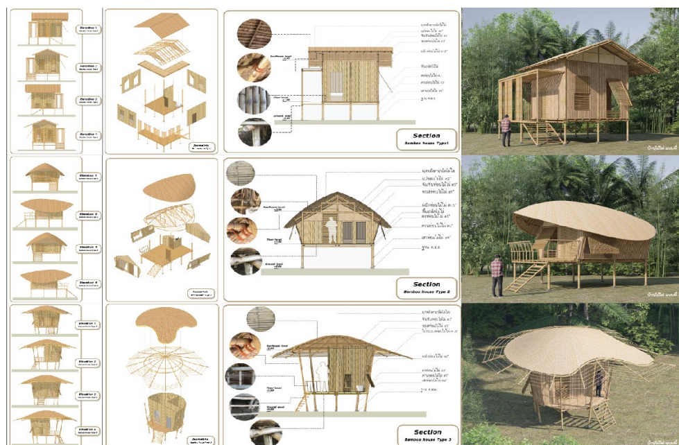
ภาพที่ 11 ผลการออกแบบบ้านไม้ไผ่ 3 แบบ ที่มีการประยุกต์ใช้ระบบ Prefabricated และ Modular
