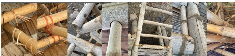
ภาพที่ 8 การเก็บข้อมูลการยึดชิ้นส่วนขององค์อาคาร
