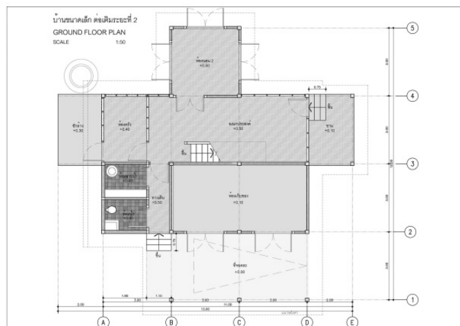
ภาพที่ 6 ผังพื้นที่ชั้นล่าง บ้านขนาดเล็ก ต่อเติมระยะที่ 2
