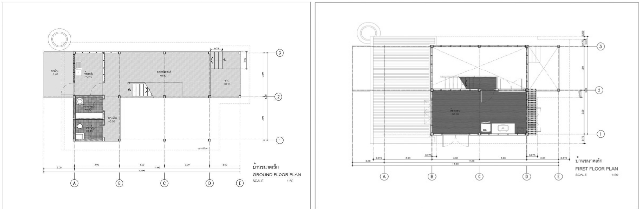
ภาพที่ 2 ผังพื้นชั้นล่าง (ซ้าย)และ ผังพื้นชั้นบน (ขวา) บ้านขนาดเล็ก
