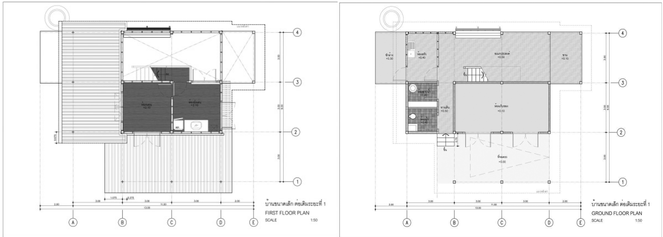
ภาพที่ 4 ผังพื้นที่ชั้นล่าง (ซ้าย)และผังพื้นที่ชั้นบน (ขวา) บ้านขนาดเล็ก ต่อเติมระยะที่ 1
