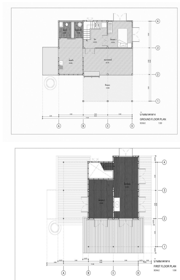
ภาพที่ 8 ผังพื้นที่ล่าง (บน) และ ชั้นบน (ล่าง) บ้านขนาดกลาง
