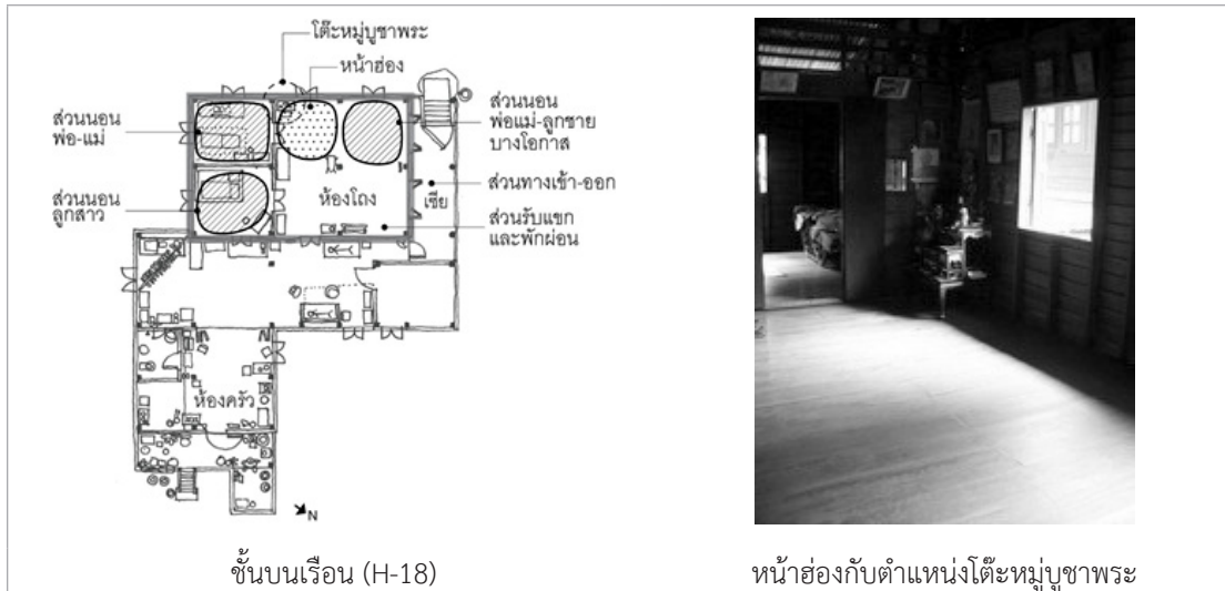
ภาพที่ 8 แสดงลักษณะการใช้งานพื้นที่ภายในของเรือนประยุกต์
