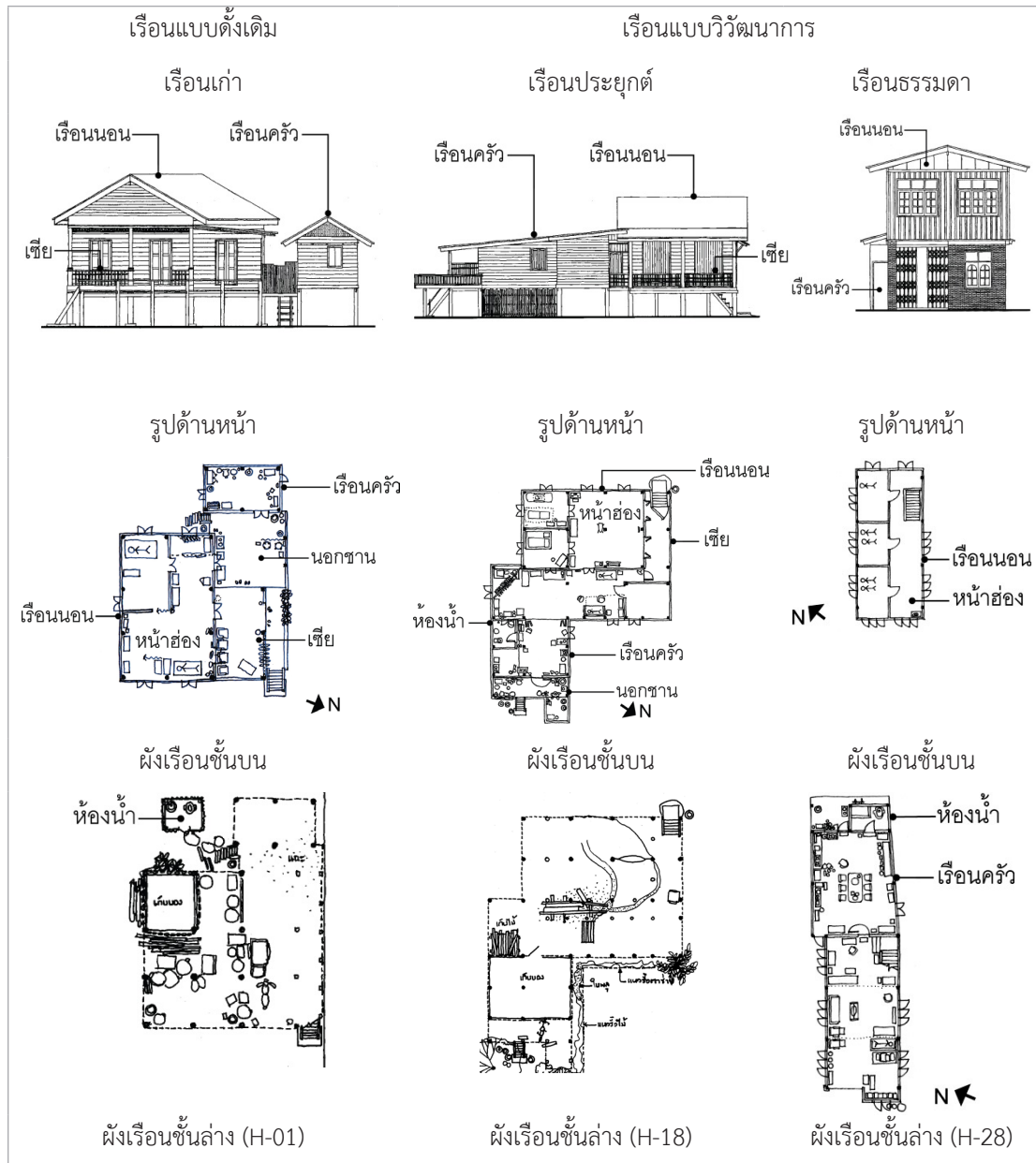
ภาพที่ 6 แสดงรูปแบบเรือนแบบดั้งเดิมและเรือนแบบวิวัฒนาการ
