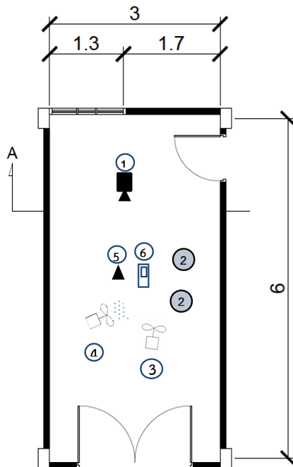
ภาพที่ 2 การติดตั้งอุปกรณ์ในห้องทดลอง หมายเลข (1) กล้องวิดีโอ (2) แก้ว (3) พัดลม (4) พัดลมไอเย็น (5) อุปกรณ์วัดความเร็วลม (6) อุปกรณ์วัดอุณหภูมิและความชื้น
