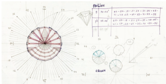
ภาพที่ 4: ผลงานออกแบบเหลื่อมเจียรไนขั้นต้นจากการเขียนแบบด้วยมืออย่างคร่าว ที่มา: สุภารีย์ เถาว์วงศ์ษา
